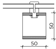
zimnogięty ceownik równoramienny 50x50x3,25 mm typ 1, pojedyncze, szt. 40, Kolor RAL 7016 matowy
