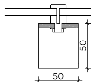
zimnogięty katownik równoramienny 50x50x3,25 mm typ 2, podwójne, szt. 10. Kolor RAL 7016, matowy.
