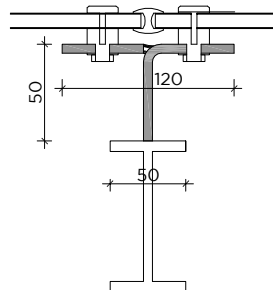
WSPORNIK POSZYCIA TYP 2, SZT. 10
