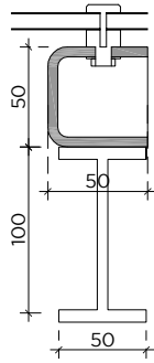
WSPORNIK POSZYCIA TYP 2, SZT. 40
