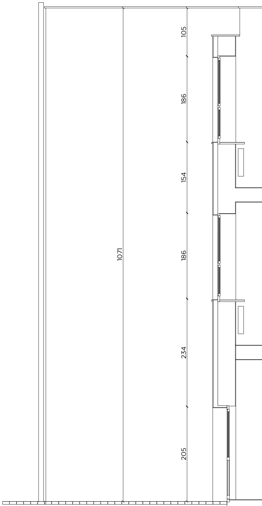
PRZEKRÓJ A-A SKALA 1:50
